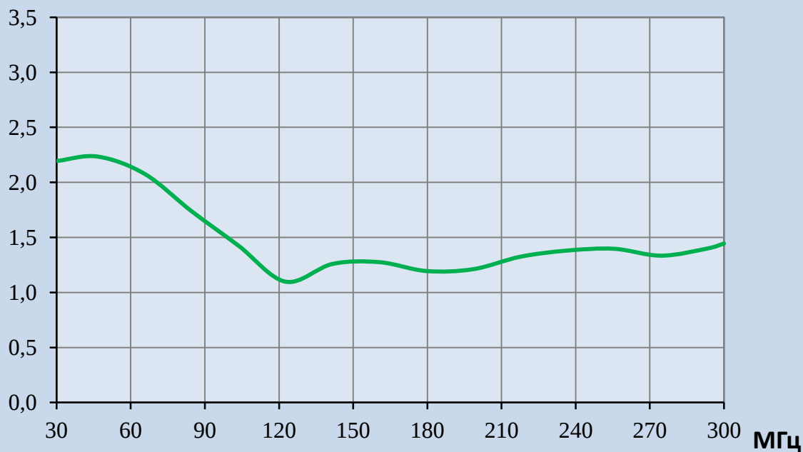
Типовое значение КСВН
