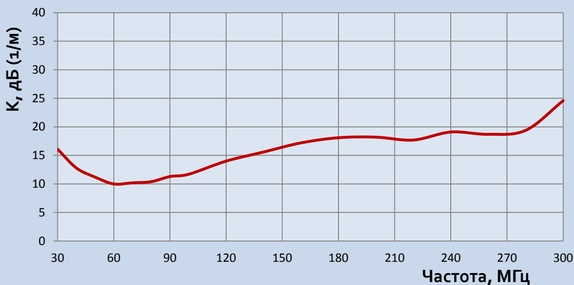
Типовой коэффициент калибровки
