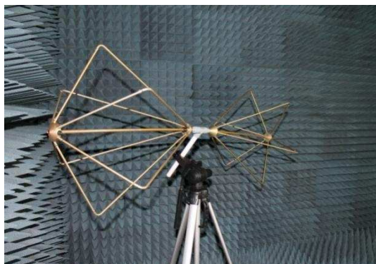
Фото 2. Антенна П6-121 на штативе, в рабочем положении
