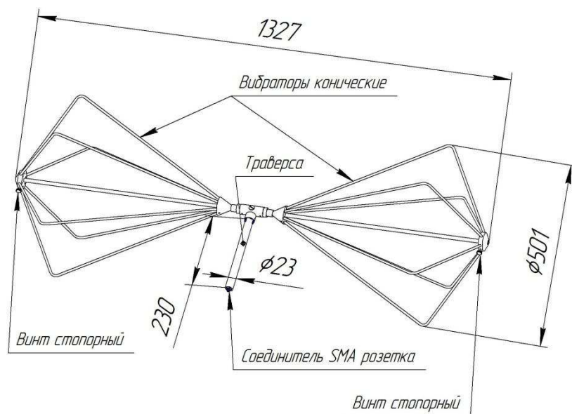
Рис.1 Габаритный чертеж антенны П6-121
