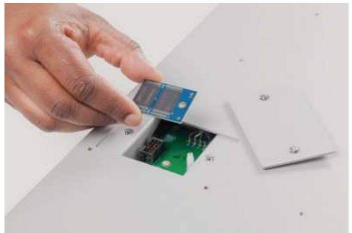
Рисунок 8. Установка «черного ящика» N7908A BBR в источник питания APS
