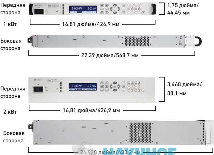
Рисунок 12. Источники питания мощностью 1 и 2 кВт, размеры передней и боковой сторон
