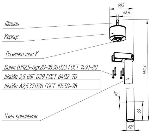
Рис.1 Габаритный чертеж антенна АС7.24
