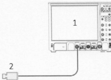
Рисунок 2 – Схема соединений при установке нуля преобразователей измерительных N1921A и N1922A
