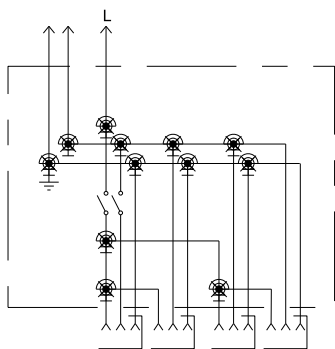
1. АЛ(Ф)-ЭПА стандартная с выключателем
