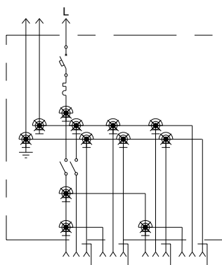
2. АЛ(Ф)-ЭПА с выключателем и автоматом безопасности
