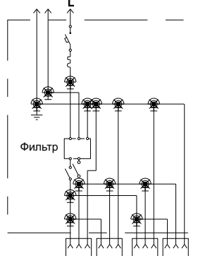
6. АЛ(Ф)-ЭПА с выключателем, автоматом безопасности, УЗО и модулем подавления сетевых импульсов
