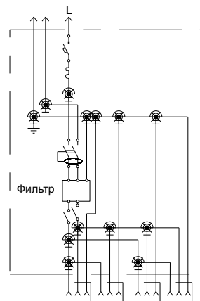
7. АЛ(Ф)-ЭПА с выключателем, устройством защитного отключения УЗО и модулем подавления сетевых импульсов
