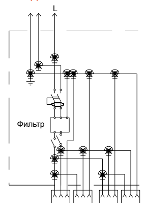
7. АЛ(Ф)-ЭПА с выключателем, устройством защитного отключения УЗО и модулем подавления сетевых импульсов
