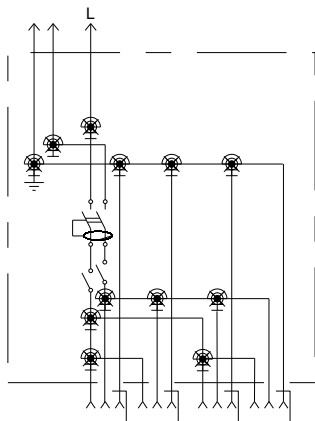
3. АЛ(Ф)-ЭПА с выключателем и устройством защитного отключения УЗО
