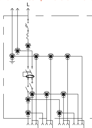
4. АЛ(Ф)-ЭПА с выключателем, автоматом безопасности и устройством защитного отключения УЗО
