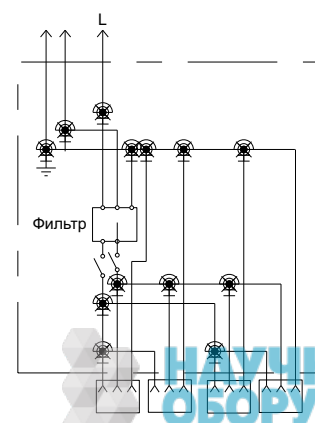
8. АЛ(Ф)-ЭПА с выключателем и модулем подавления сетевых импульсов
